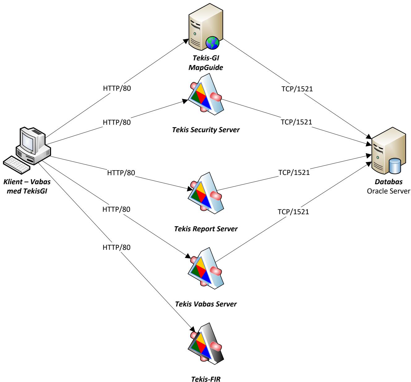
Figur 2 - Kommunikationer när Vabas med TekisGI Webb används
