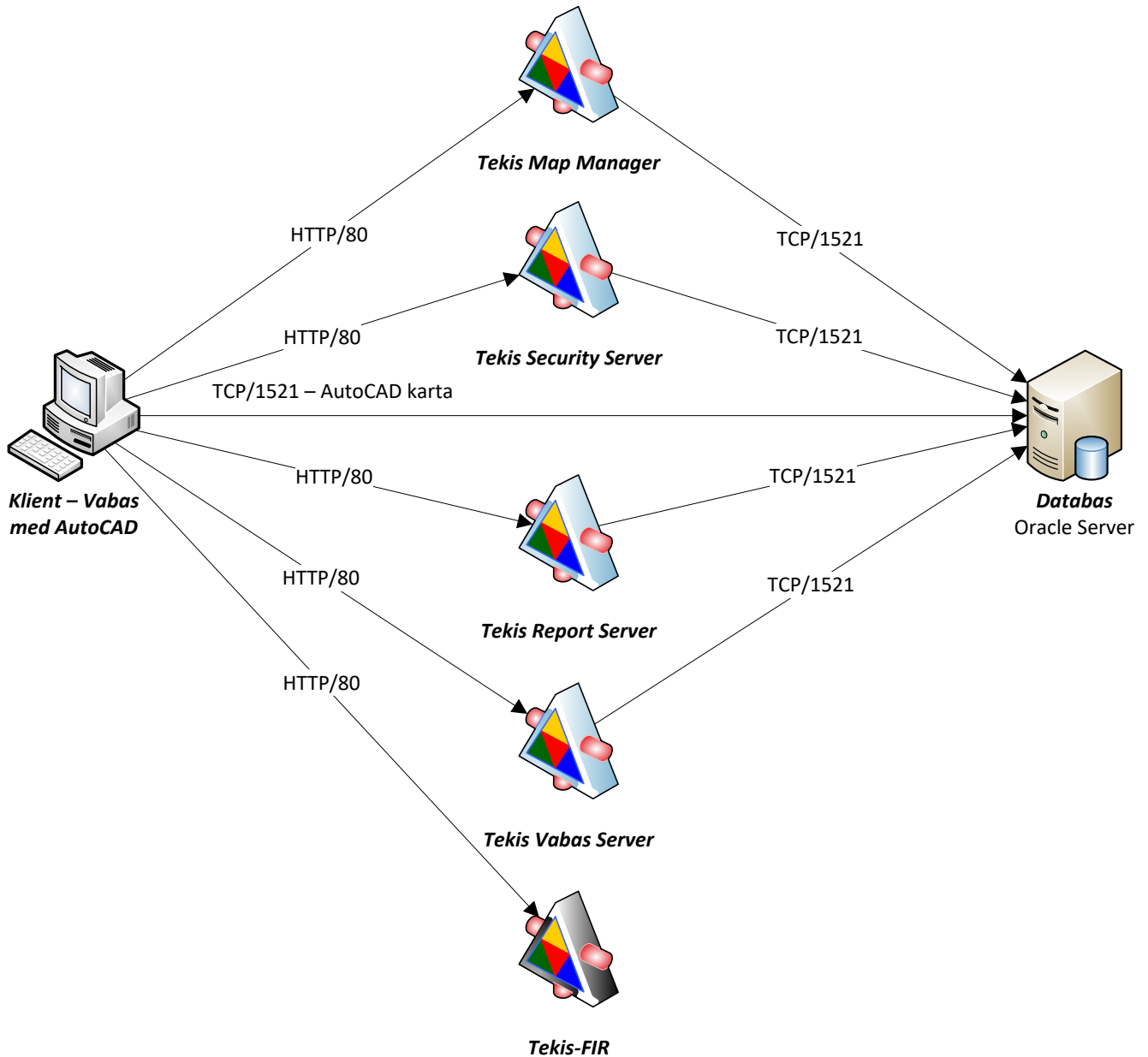
Figur 1 - Kommunikationer när Vabas för AutoCAD används
